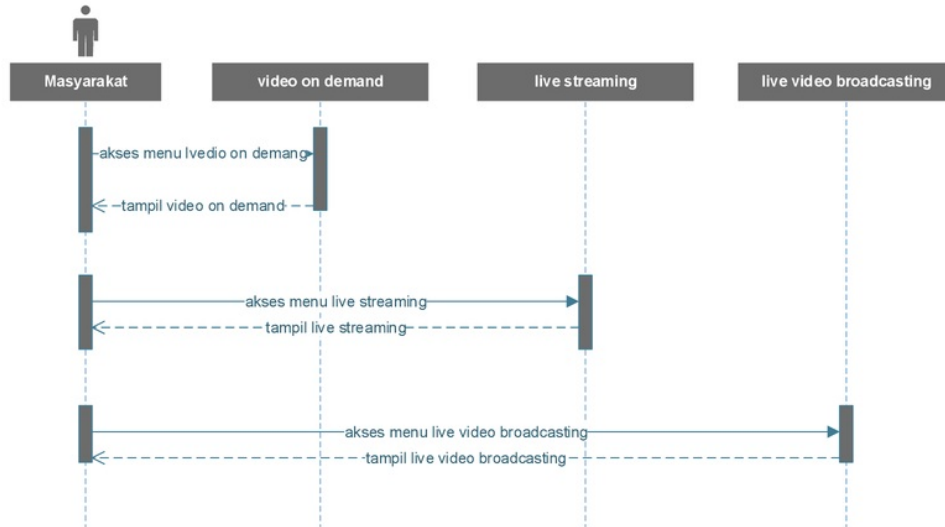
Gambar 5. Sequence Diagram Masyarakat (Pengguna)
