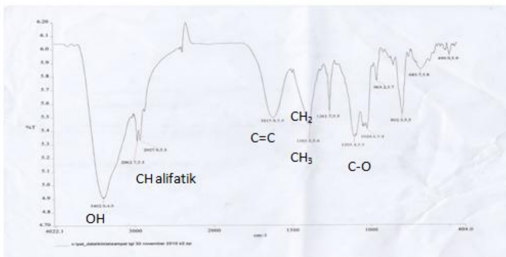
Gambar 8. Spektra Infra Merah (KBr) isolat batang Alsophila glauca J.Sm
