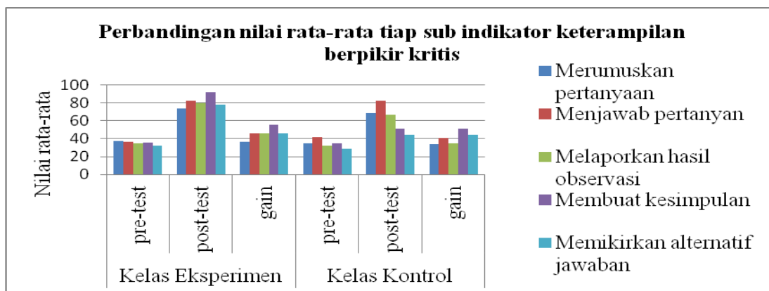
Diagram 2. Perbandingan Nilai Rata-Rata Pre-test , Post-test dan Gain Tiap Sub Indikator Keterampilan Berpikir Kritis
