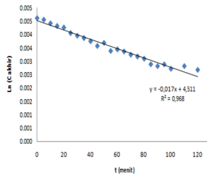
Gambar C.2 Grafik kinetika reaksi orde satu pada elektrodekolourisasi remazol violet 5R
