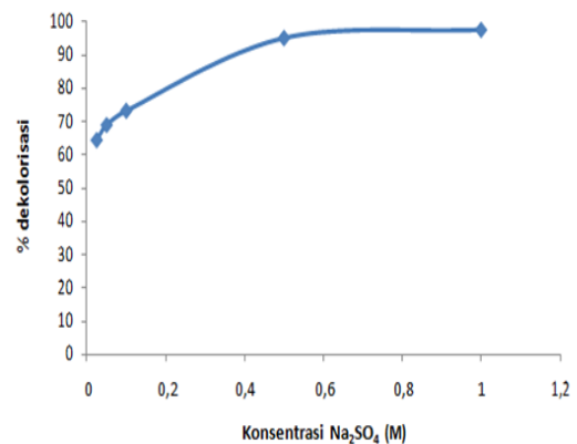
Gambar C.3 Grafik hubungan % dekolourisasi dan konsentrasi Na 2 SO 4 pada elektrodekolourisasi remazol violet 5R
