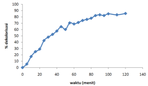
Gambar C.1 Grafik hubungan % dekolourisasi terhadap waktu elektrolisis
