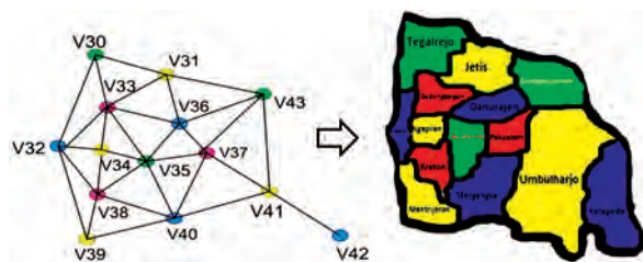
Gambar 7. Hasil pewarnaan graf dan alternatif peta kotamadya Yogyakarta
