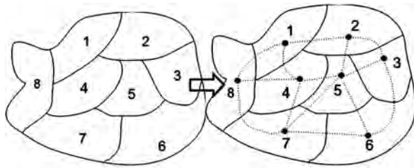
Gambar 3. Peta M dan Graf Dual G^*
