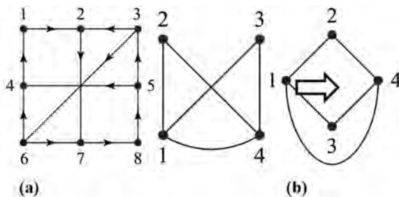
Gambar 2. (a) Graf berarah (b) Sirkuit elektrik
