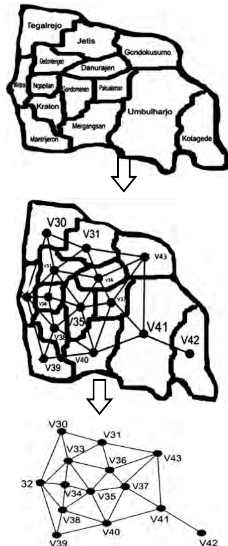
Gambar 6. Peta kotamadya Yogyakarta beserta dengan graf dualnya
