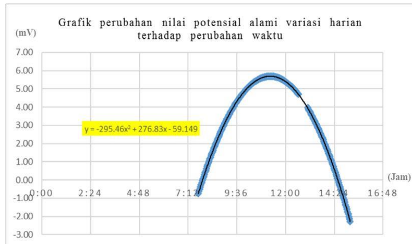
Gambar 6. Grafik waktu terhadap nilai variasi harian (a) Grafik area A (b) Grafik area B
