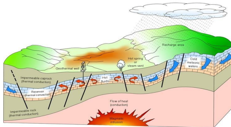
Gambar 2. Skema Sebuah Sistem Geotermal yang Ideal [4]
